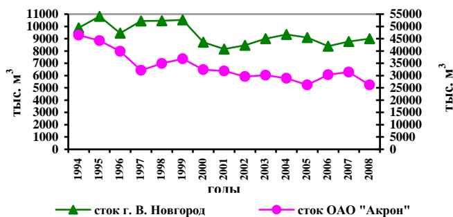
Динамика поступления сточных вод на биологические очистные сооружения
